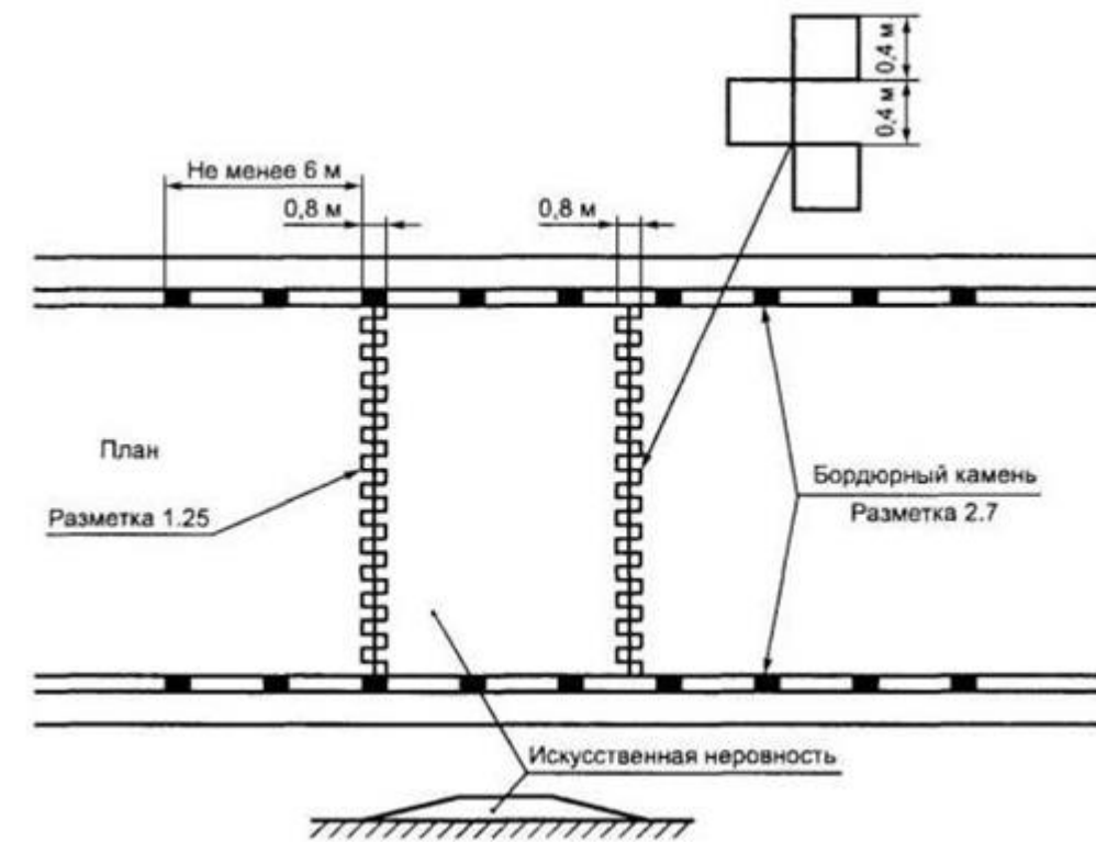
Рисунок 11 - сборно-разборная конструкция
